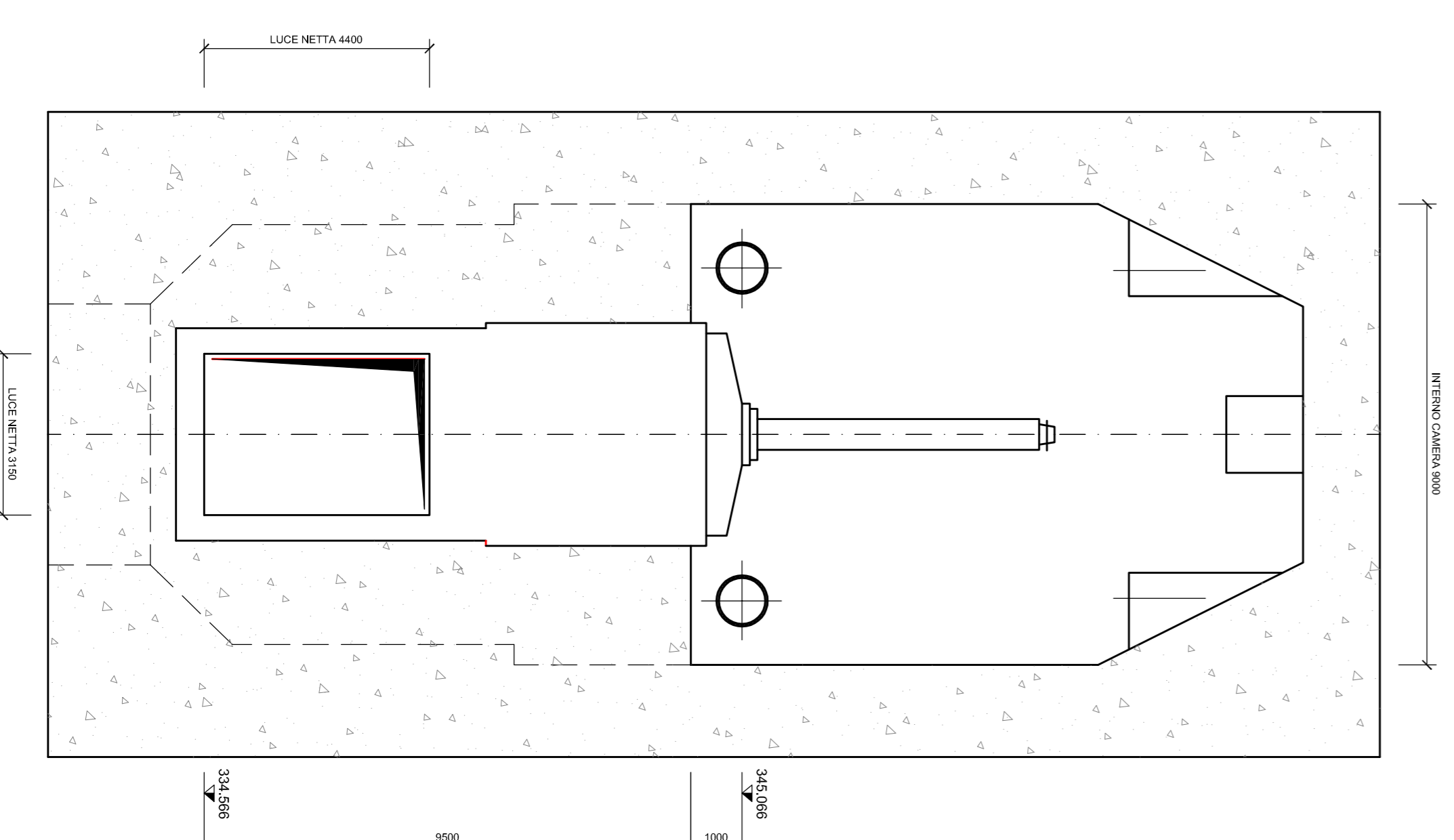
SEZIONE B-B 1:100
